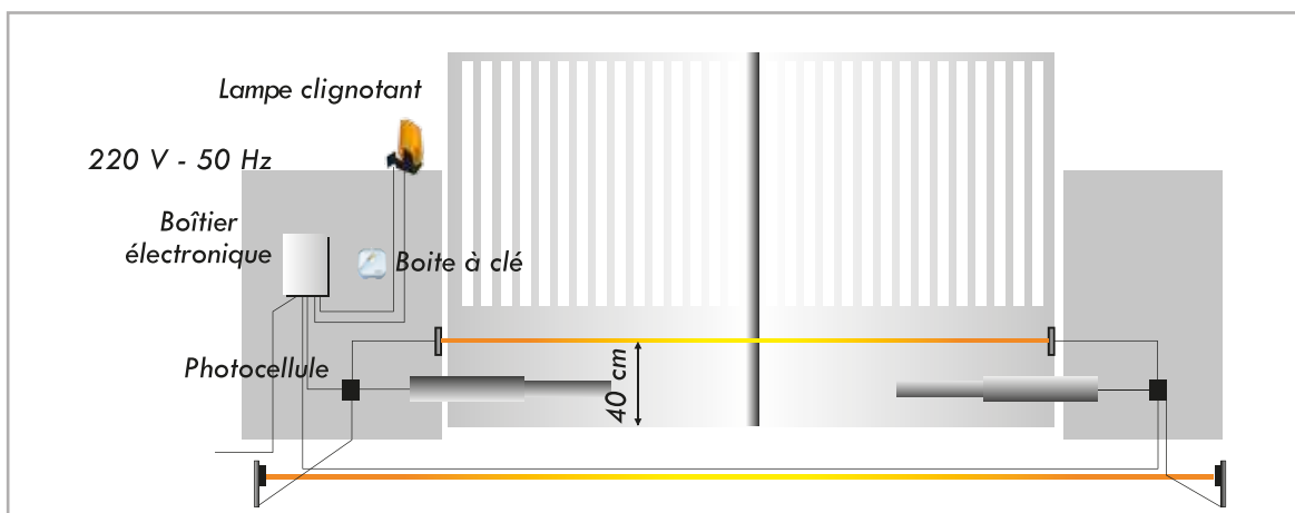
Schéma de détails techniques d'une porte battante
