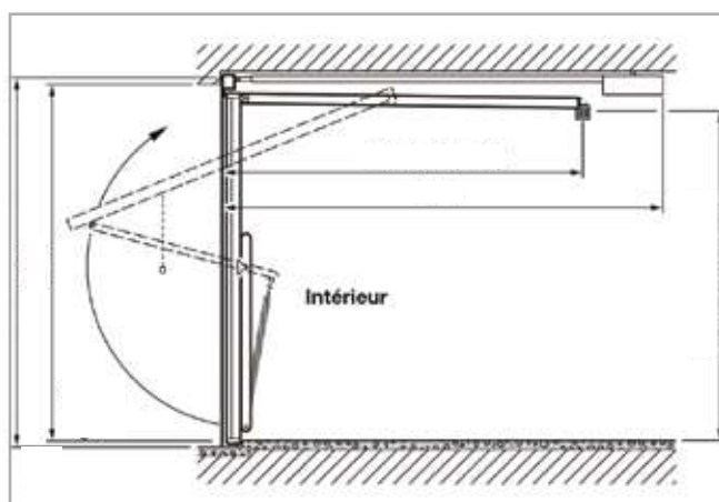
Porte de garage basculante débordante
