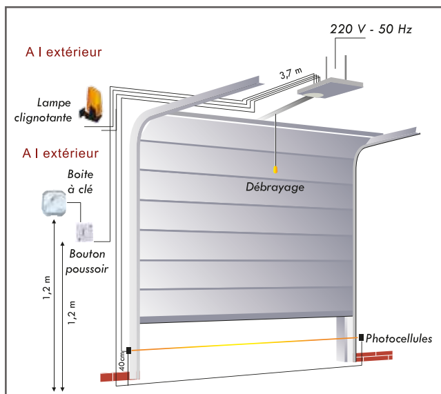
Porte Sectionnelle
