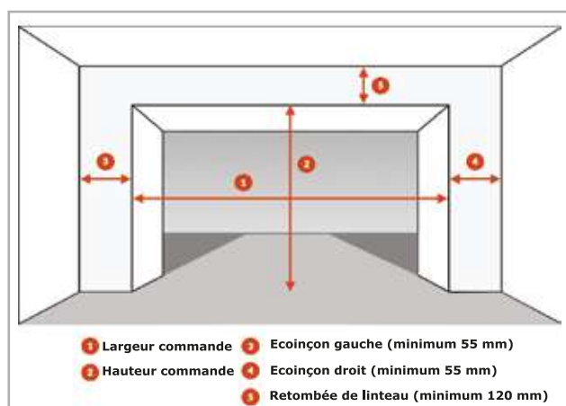
Prise de mesures pour porte de garage basculante
