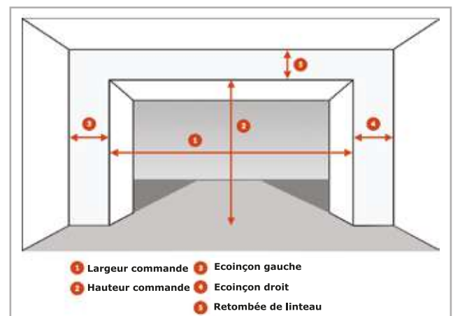
Prise de mesures pour porte de garage Sectionnelle
