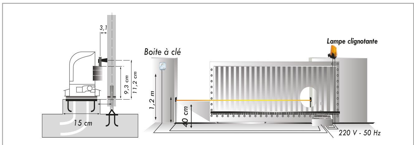
Schéma de détails techniques d'une porte coulissante
